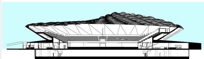
SEZIONE TRASVERSALA SC. 1/100
